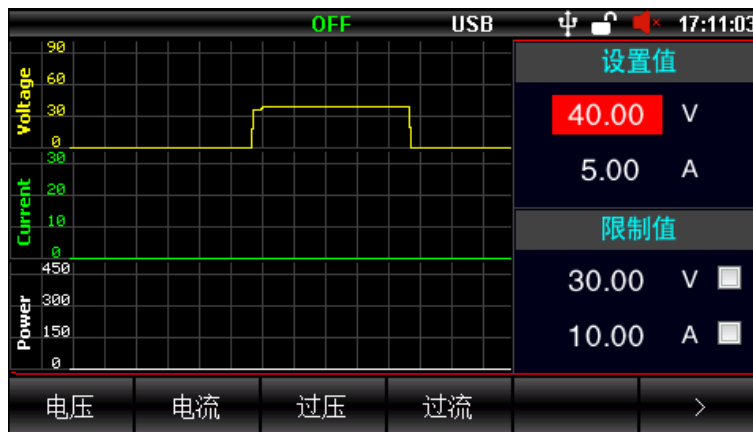
图 12-1 波形显示
