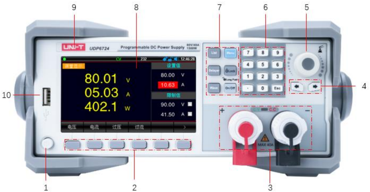
图 4-1 直流电源前面板
