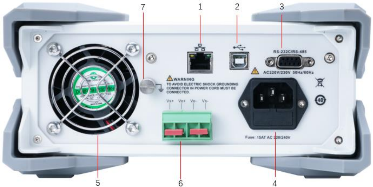
图 4-2 直流电源后面板
